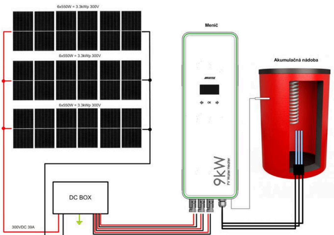
Základní blokové schéma samostatné jednotky
